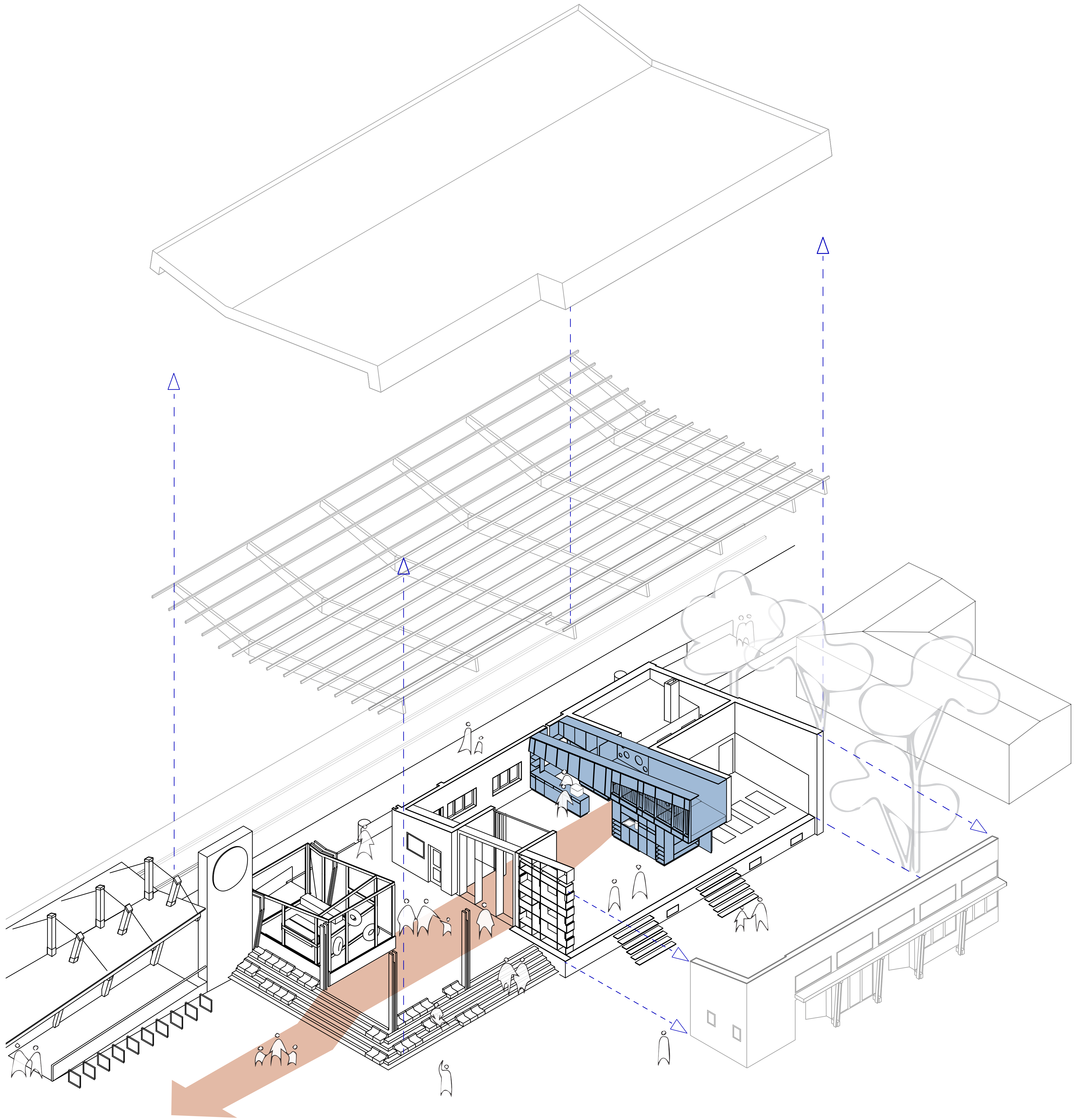
Explosionszeichnung Landungsplatz 8
