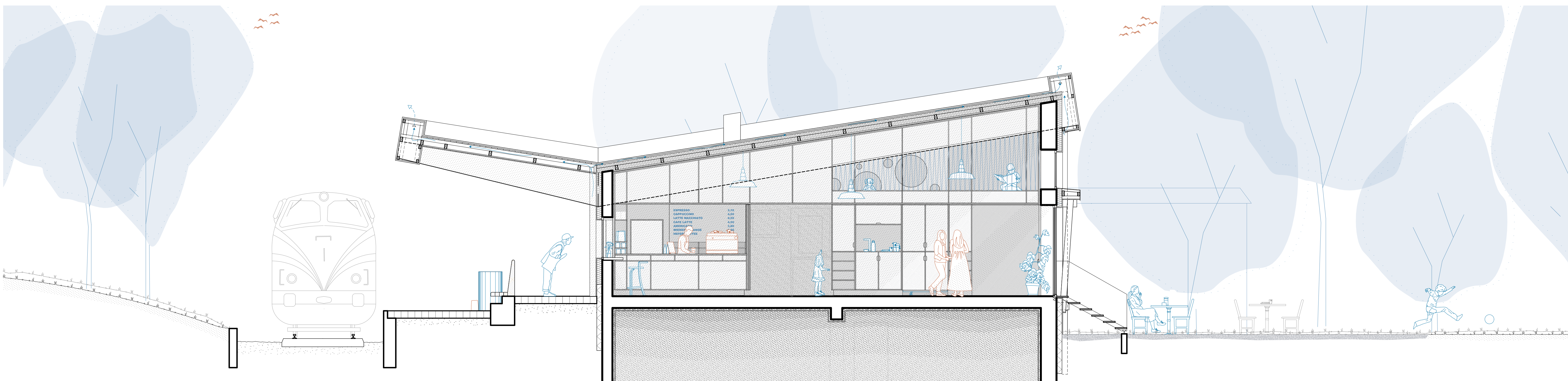
Querschnitt Landungsplatz M1:50 12
