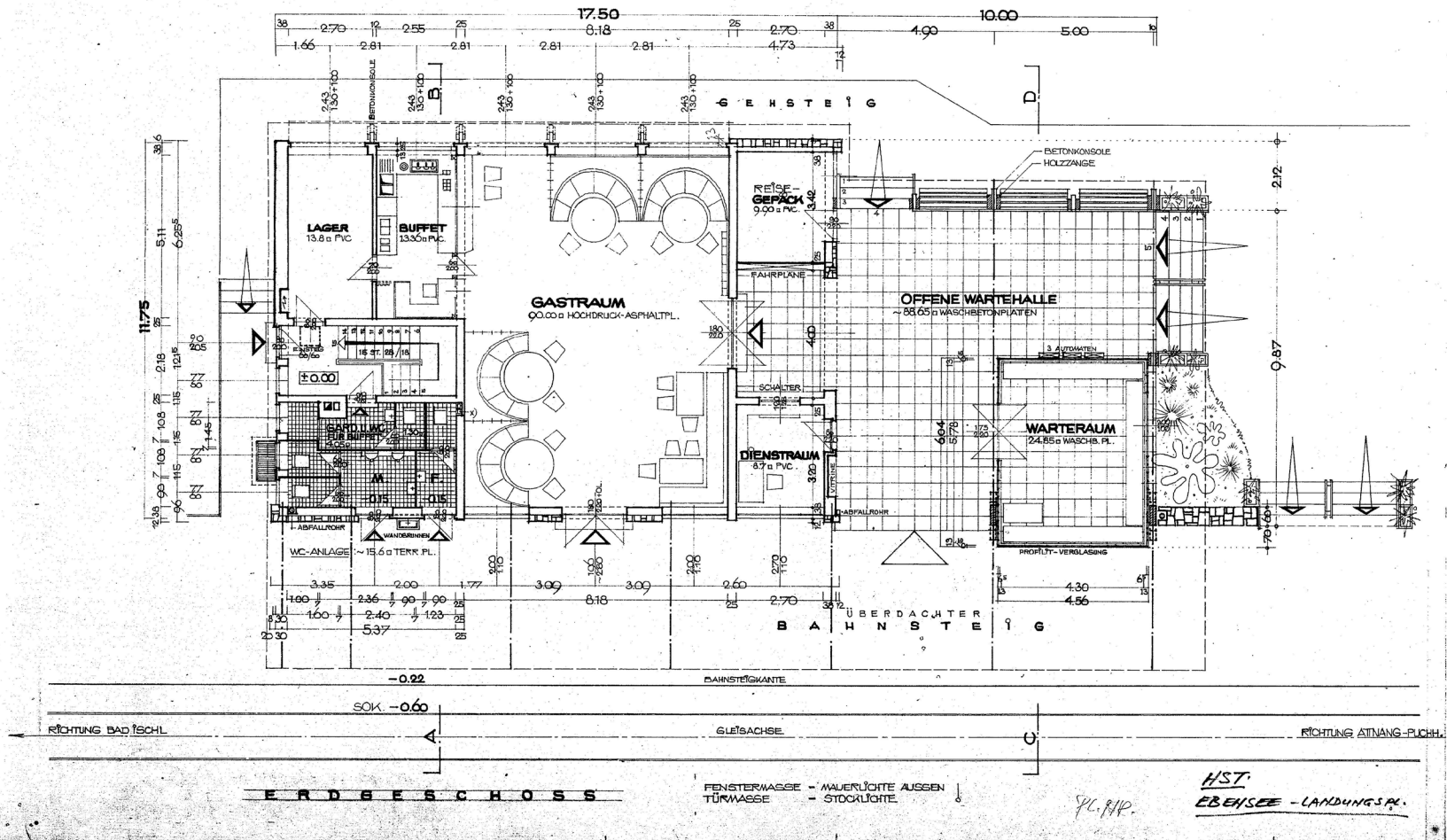
ÖBB Hst Ebensee Ldpl. - Lageplan Gast-, Warte-, Dienstraum von 1970; ÖBB
