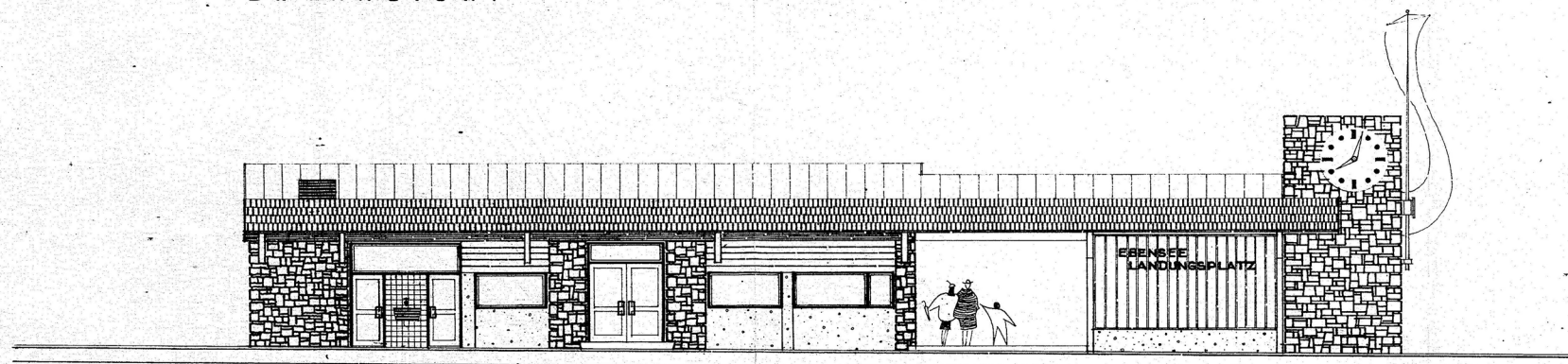
NO ANSICHT (GLEISSEITIG)
