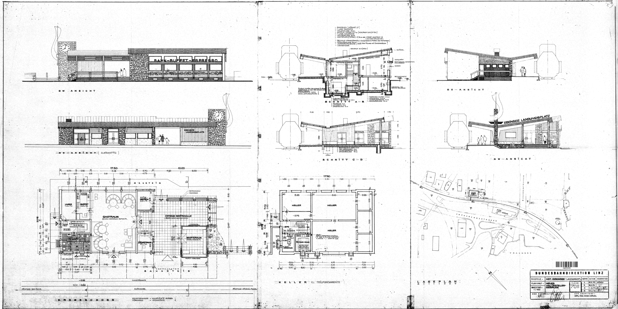
ÖBB Hst Ebensee Ldpl - Grundrisse Ansichten Lageplan von 1970
